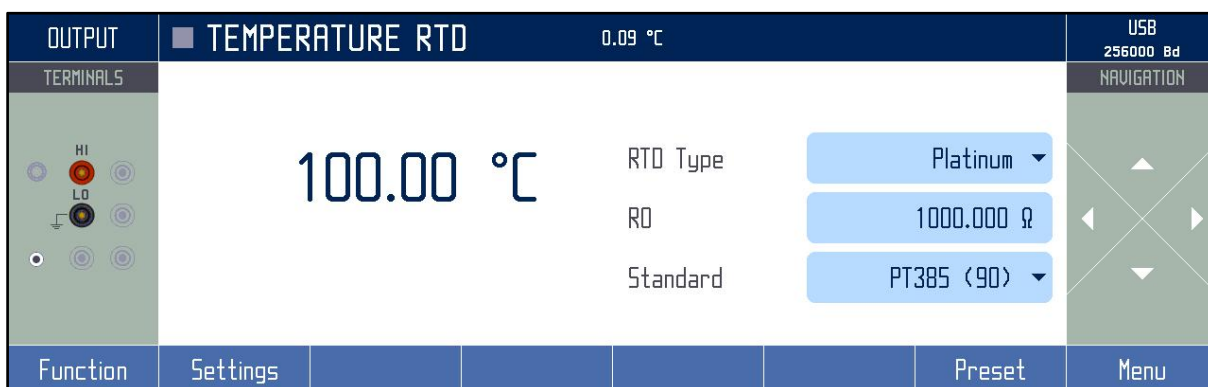
Obr. 31 Simulace odporových teplotních snímačů RTD
