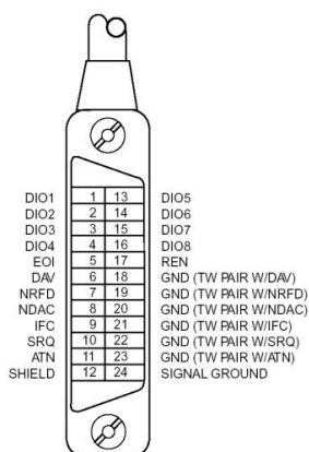
Obrázek 22 Konektor GPIB
