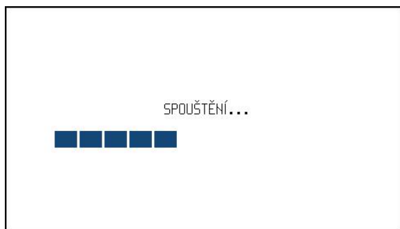
Obrázek 1 Úvodní obrazovka
