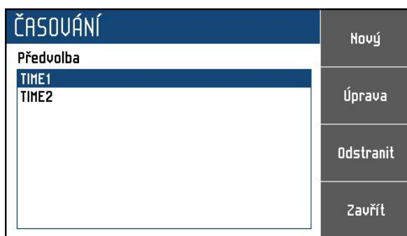
Obrázek 12 Seznam sekvencí
