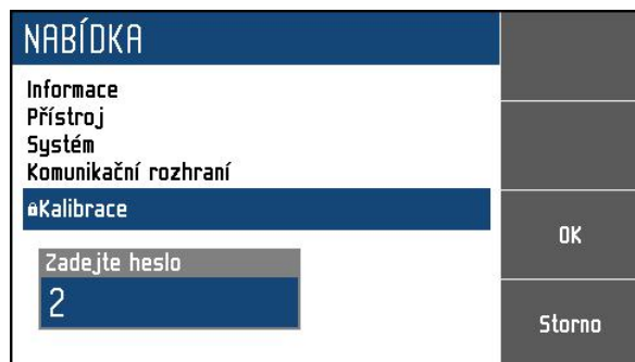
Obrázek 18 Zadání hesla
