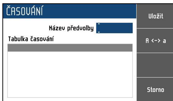
Obrázek 13 Nová sekvence
