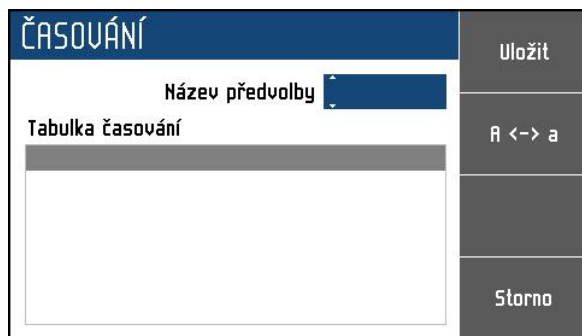
Obrázek 13 Nová sekvence
